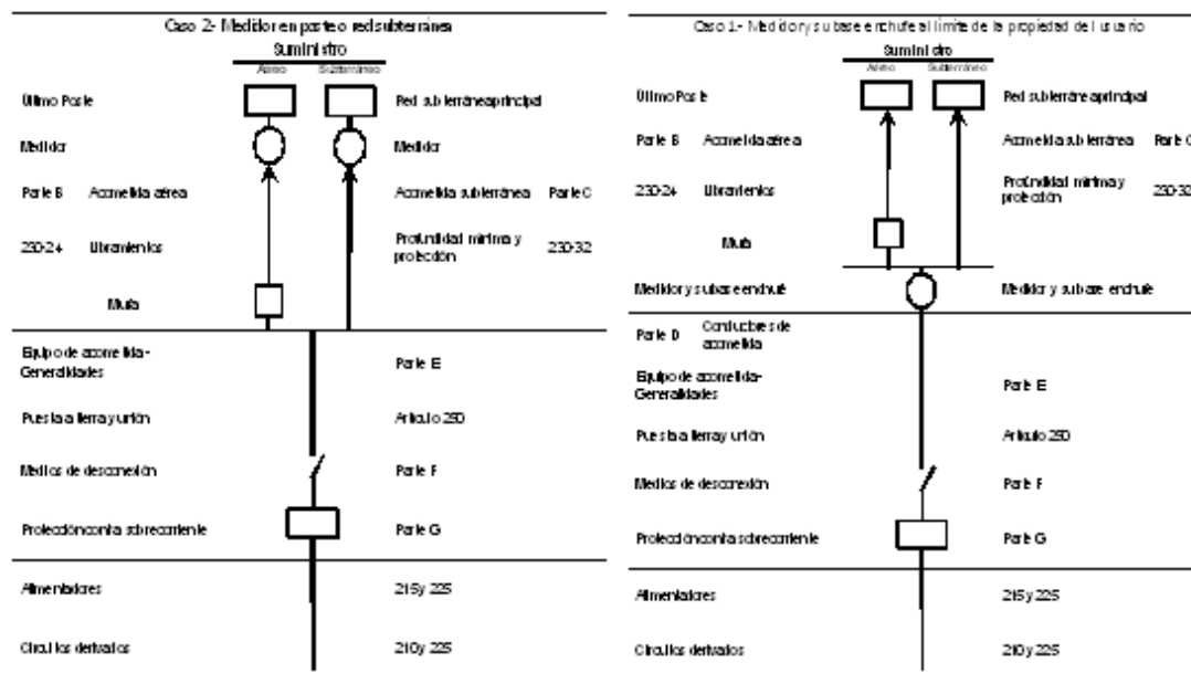
Figura 230-1.- Acometidas
